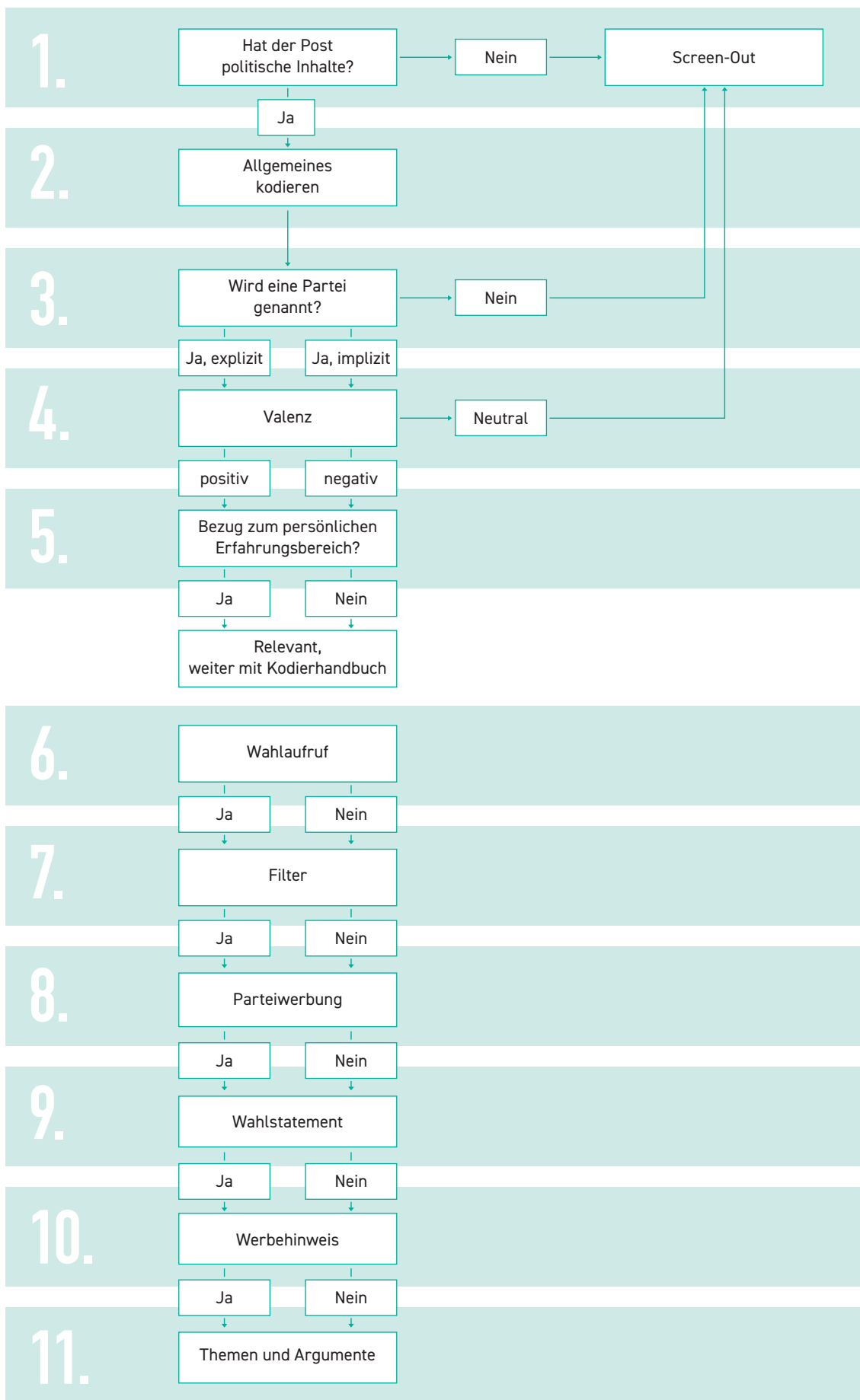
Abbildung 3: Übersicht Kodierhandbuch
